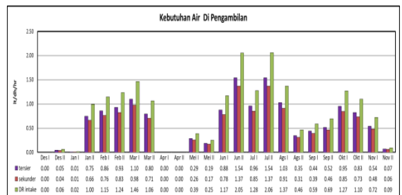
Gambar 1. Grafik kebutuhan air di pengambilan
